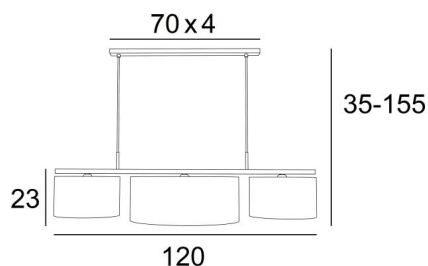
SVEND in geborsteld brons met lampenkappen in Raphia Banane en Raphia Nature (materialen uit categorie 3)
