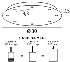
CEILING BASE 8 o30 en bronze léger (option). Finition du métal : code 28. En option : un grand choix de câbles et de douilles (+supplément)
