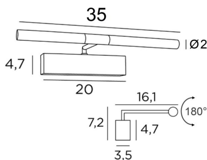
MEIDOUUM 35 en laiton (poli et satiné). Finition du métal : code 20
