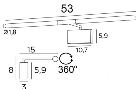
MEROE 53 en nickel satiné. Finition du métal : code 33
