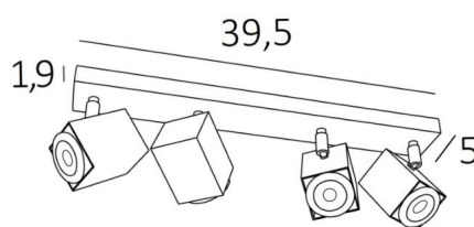
MAJORIS 4 in gebürstet Bronze. Metalloberfläche Code: 29
