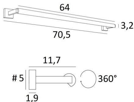
CREMONE 65 in gebürstet Bronze. Metalloberfläche Code: 29
